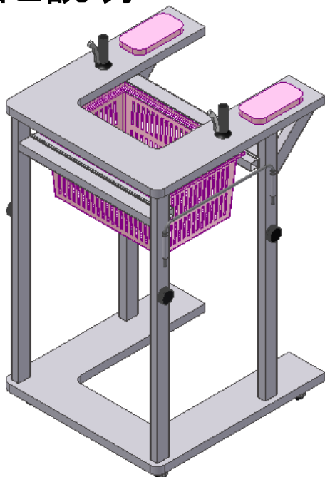
全体図
